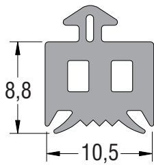
escala 2:1
