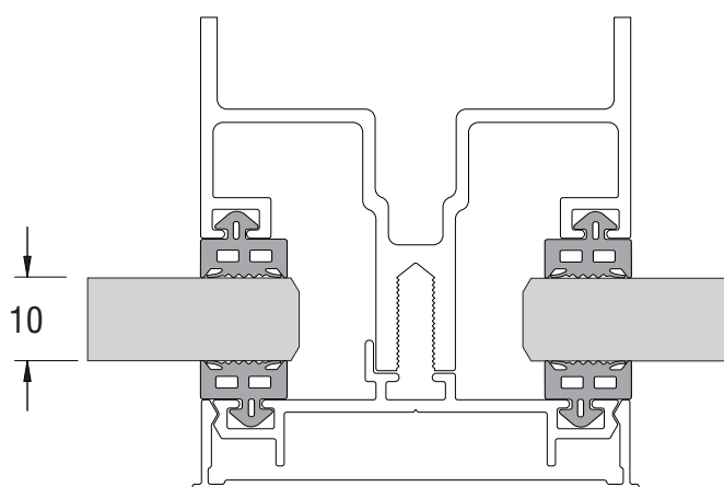
escala 1:1
