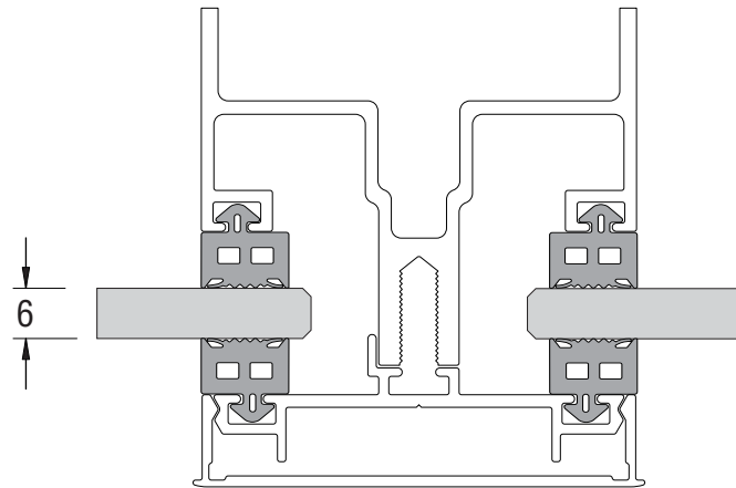
escala 1:1
